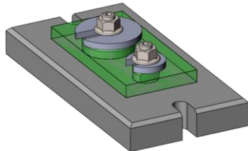
Prise de pièce en montage centrage-locating
