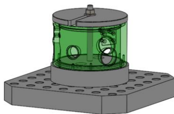
Prise de pièce centrée sur palette sur CUH
