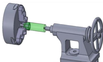
Prise de pièce en mandrin trois mors durs avec contre pointe
