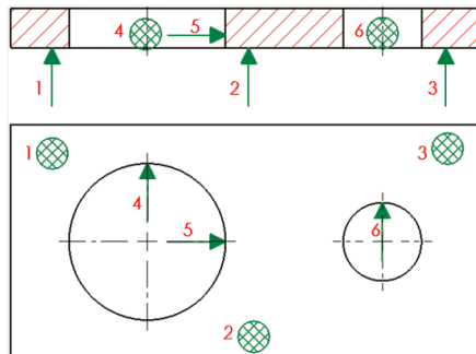
Prise de pièce en montage centrage-locating
