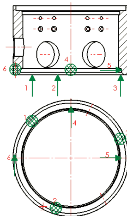
Prise de pièce centrée sur palette sur CUH
